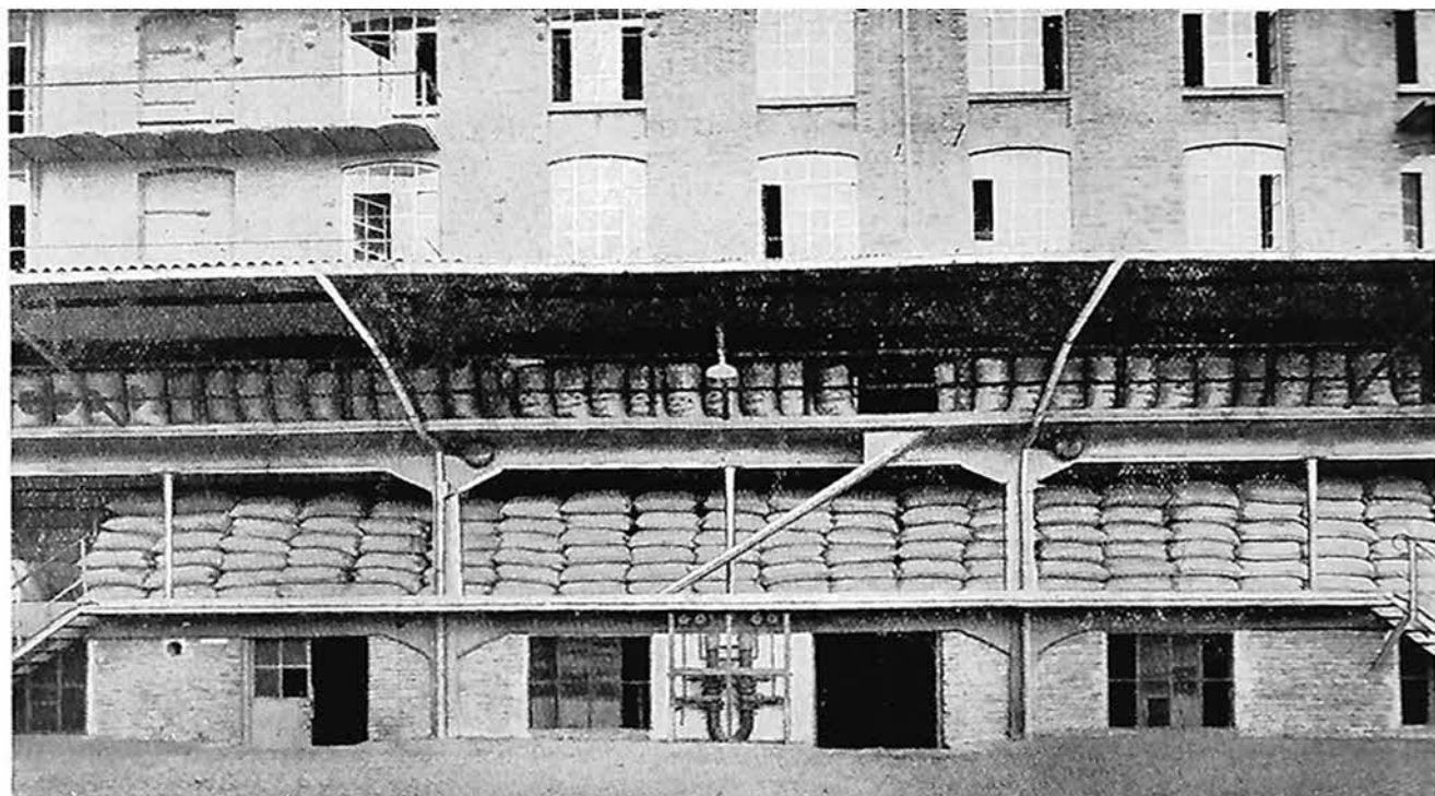
Molino interamente protetto contro l'incendio a mezzo di una installazione di estintori meccanici "GRINNELL,,
