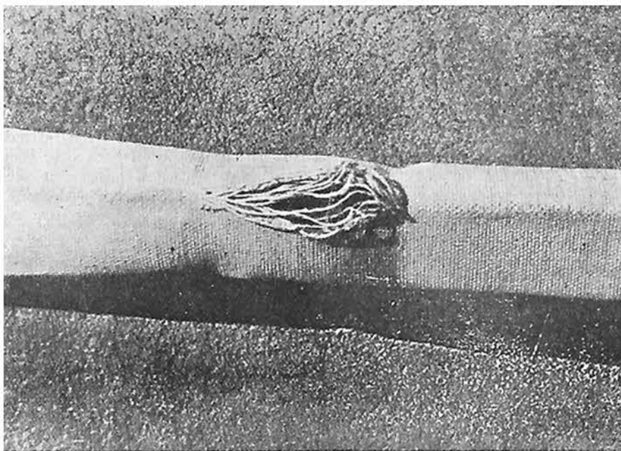
Lo scoppio avviene sempre lungo la piega e, come mostra la fotografia, tutti i fili della catena restano intatti.
