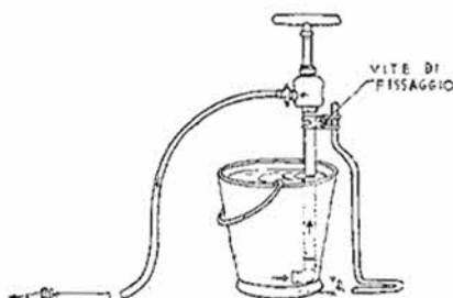
La pompa a mano casalinga di dotazione in Germania.
