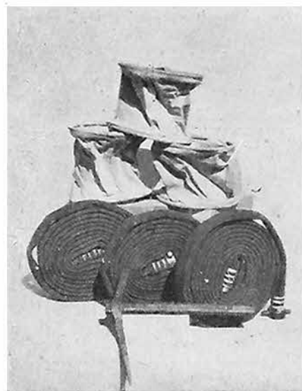
Corredo della pompa: Tre secchi di tela - Una picchetta da muratore - 18 metri di tubo tannato da m'm 25.
