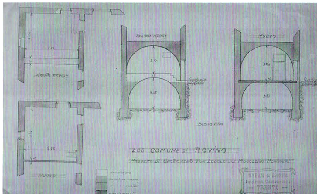
22 aprile 1914 - Progetto di adattamento di un locale ad uso magazzino Pompieri
