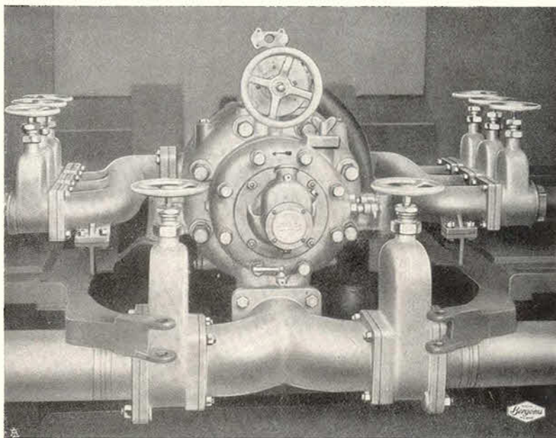
La pompa 3000/8
