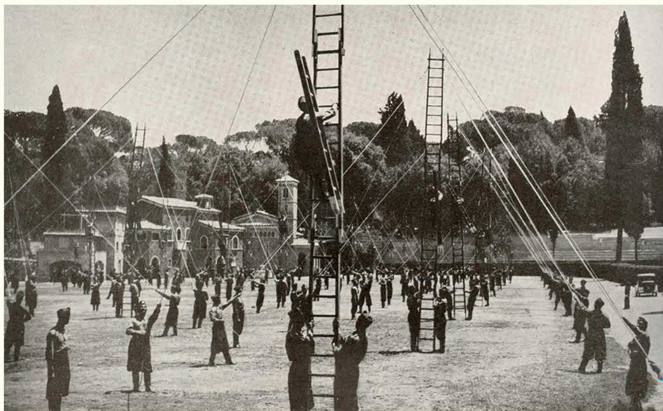
Scale italiane controventate: aggiunta della cima
